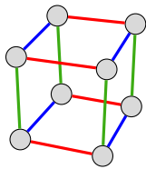
C_2 \times C_2 \times C_2
